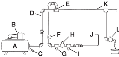
Abbeelding 1: Luchttoevoer
