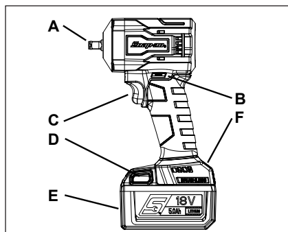
図 1: コードレスインパクトレンチ
