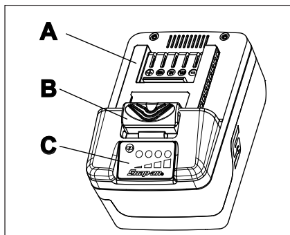
Abbildung 7: Akku (CTB8187)
