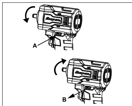
図 3: 正逆切替スイッチ
