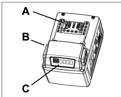
Figure 5 : Bloc-batterie (CTB185/CTB1856)
