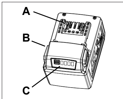
Abbildung 5: Akku (CTB185/CTB1856)
