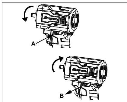
Abbildung 3: Vorwärts-/Rückwärtsschalter
