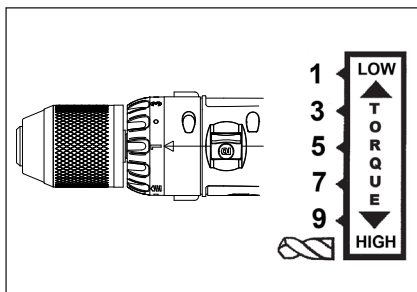
Abbildung 2: Drehmoment-Einstellring
