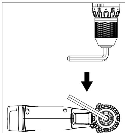
図 5: チャックを緩める
