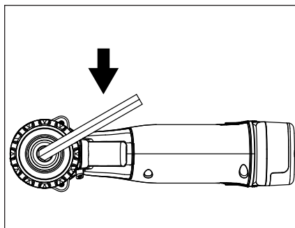
Figura 6: Serraggio del mandrino
