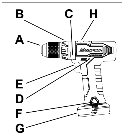
図 1: コードレスドリル
