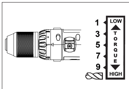
Afbeelding 2: Koppelinstelling
