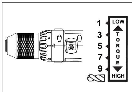
Figura 2: Ghiera di regolazione della coppia di serraggio
