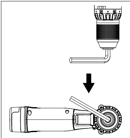
Abbildung 5: Lösen des Spannftters
