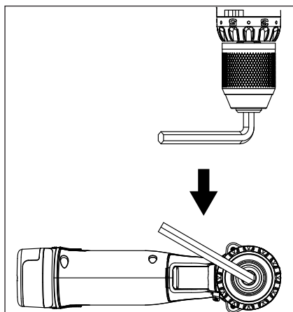
Figure 5 : Desserrage du mandrin
